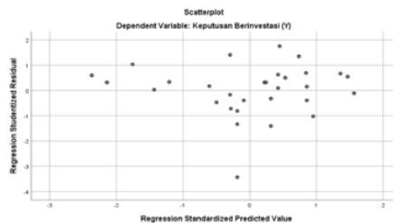
Gambar 4.1 Uji Heteroskedastisitas
