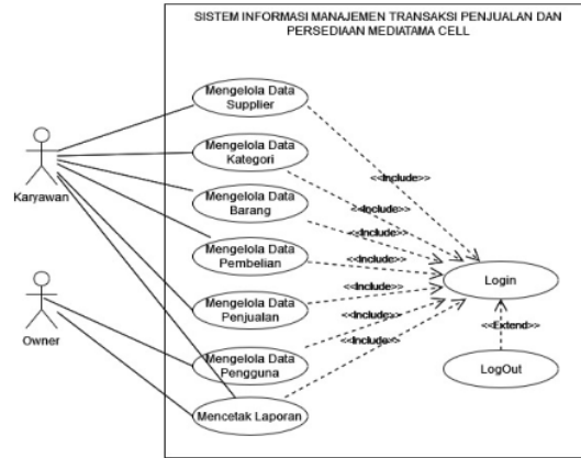
Gambar 2. Use Case Diagram Transaksi Penjualan dan Persediaan Mediatama
